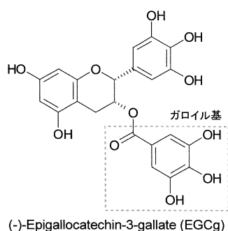
Fig. 2 エピガロカテキンガレート (EGCg) の化学構造式
